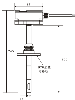
法兰安装型
