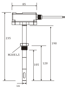
密封螺纹型
